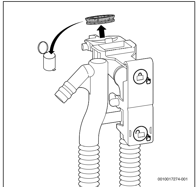
Мал. 59 Заміна ущільнення у верхній частині сифона для відведення конденсату
