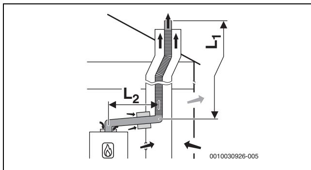
Мал. 18 Система відведення димових газів гнучкої конструкції у шахті згідно з V_{53p} з подачею у прилад повітря з приміщення та трубопроводом з однією стінкою для відведення відпрацьованих газів у котельному приміщенні; вентиляційний отвір у шахті
