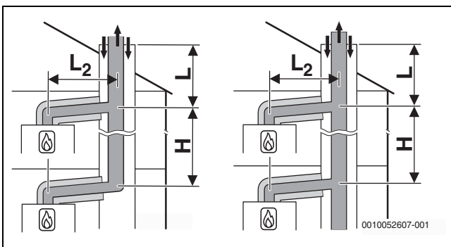
Мал. 21 Підключення декількох пристроїв згідно з C_{(14)3x} із збіркою системою відведення димових газів жорсткої конструкції і концентричною системою транспортування
