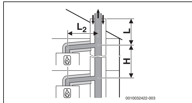
Мал. 22 Підключення декількох пристроїв згідно з C_{(14)3x} із збіркою системою відведення димових газів жорсткої конструкції і концентричною системою транспортування повітря для горіння та відпрацьованих газів у котельному приміщенні
