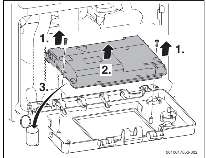
Мал. 73 Зняття корпусу та заміна друкованої плати
