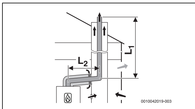
Мал. 16 Система відведення димових газів у шахті жорсткої конструкції згідно з V_{53p} з подачею повітря з приміщення через концентричний з'єднувальний трубопровід у котельному приміщенні; вентиляційний отвір у шахті
