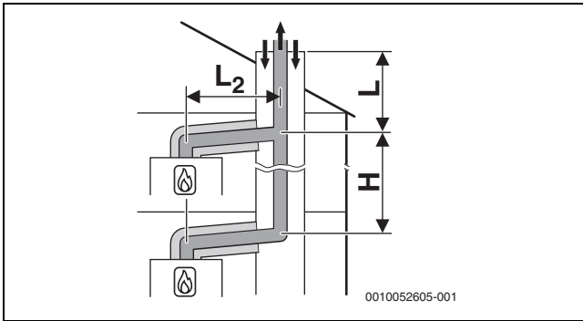
Мал. 20 Підключення декількох пристроїв згідно з C_{(14)3x} із збіркою системою відведення димових газів жорсткої конструкції і концентричною системою транспортування повітря для горіння та відпрацьованих газів у котельному приміщенні
