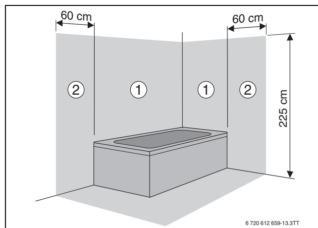
Мал. 32 Захисні зони
