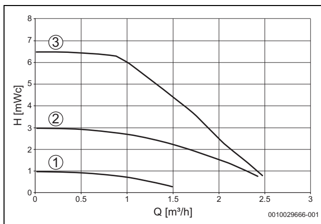
Мал. 40 Характеристична крива насоса опалювального контуру (постійний тиск)
