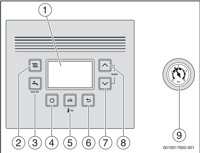
Мал. 36 Огляд панелі керування
