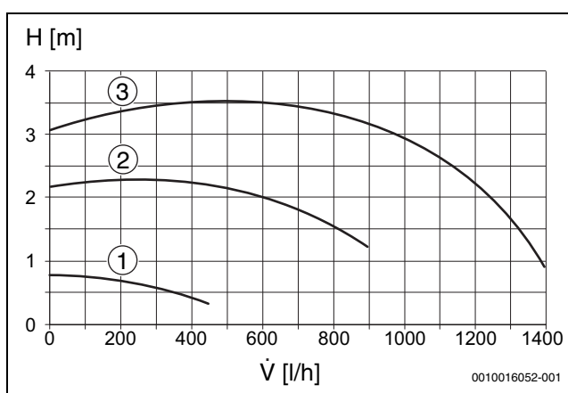
Мал. 41 Характеристична крива насоса опалювального контуру (пропорційний тиск)
