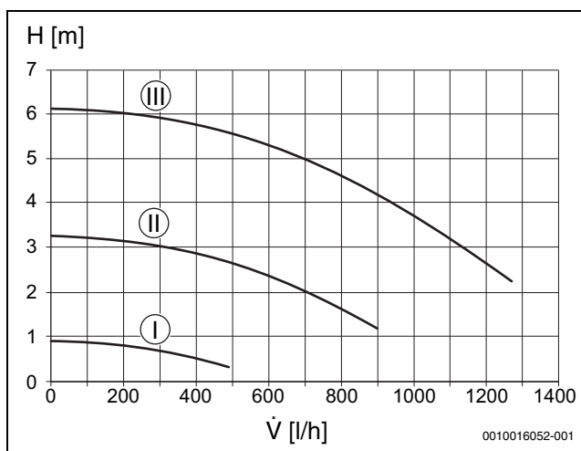
Мал. 39 Характеристична крива насоса опалювального контуру (постійна частота обертання)
