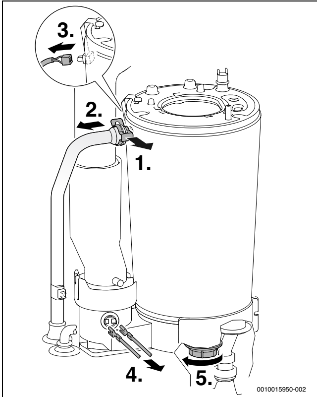
Мал. 71 Від'єднання труби лінії подачі та зняття кабелю
