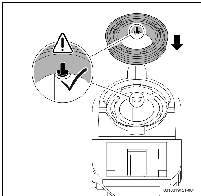
Мал. 60 Вирівнювання нового ущільнення на сифоні для відведення конденсату
