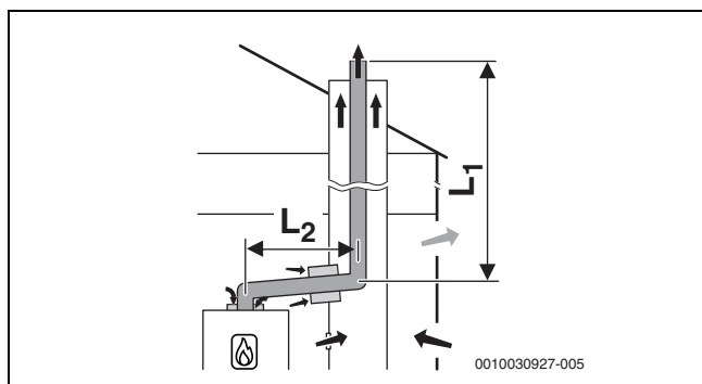
Мал. 17 Система відведення димових газів у шахті жорсткої конструкції згідно з V_{53p} з подачею у прилад повітря з приміщення та трубопроводом з однією стінкою для відведення відпрацьованих газів у котельному приміщенні; вентиляційний отвір у шахті
