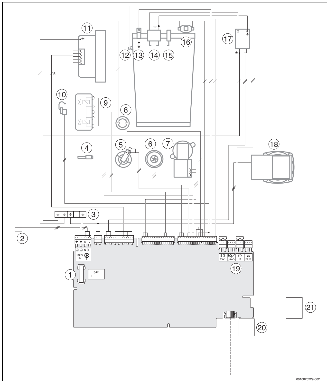
Мал. 78 Електричні підключення
