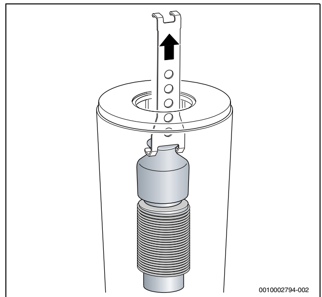
Мал. 52 Виймання верхнього елемента теплообмінника, що служить для оптимізації розподілювання тепла
