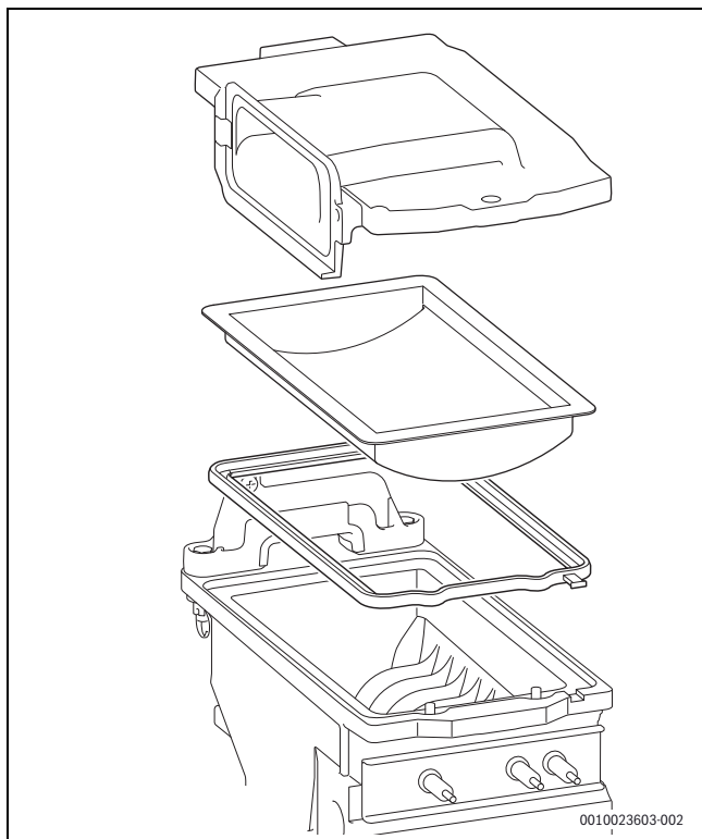
Мал. 52 Пальник
