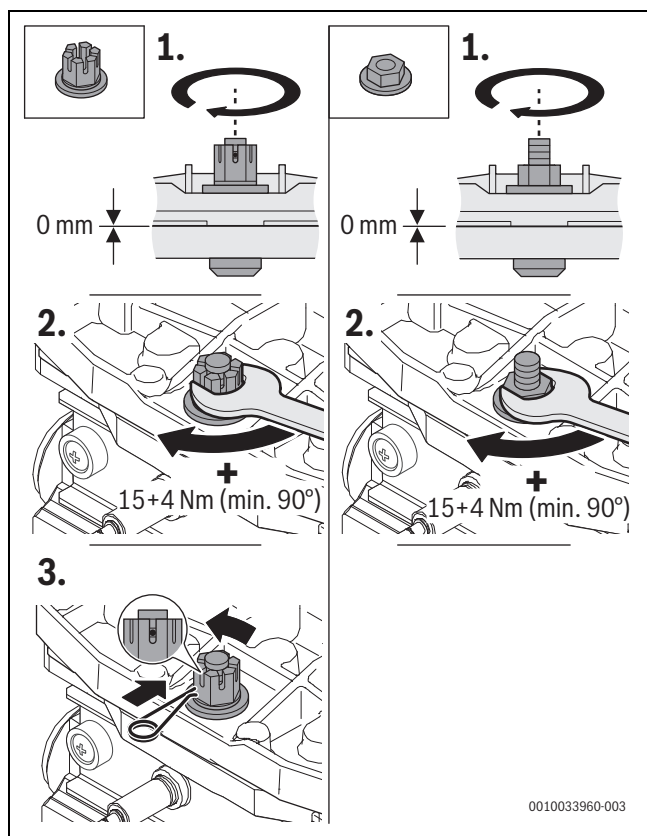
Мал. 53 Затягування гайки на кришці пальника
