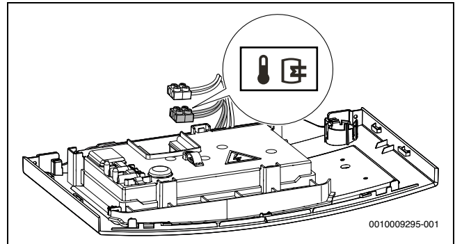
Мал. 32 Підключення датчика температури бака-водонагрівача
