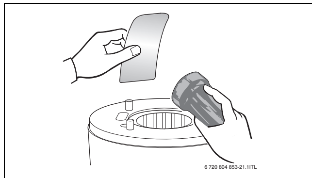
Мал. 52 Перевірка котлового блоку, який включає камеру згоряння і теплообмінник, на наявність відкладень
