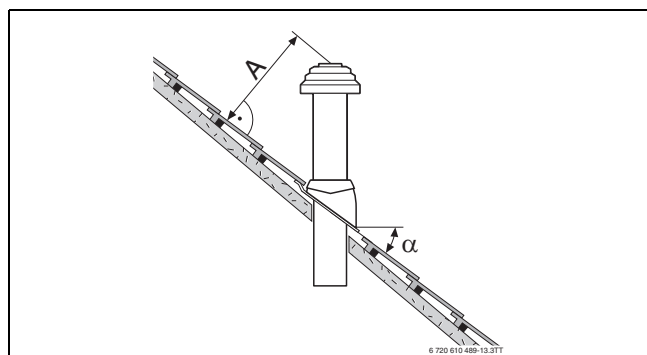
Мал. 6 Розміри відстаней і ухилів покрівлі для похилого даху
