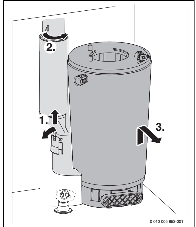
Мал. 66 Демонтаж котлового блока, який включає камеру згоряння і теплообмінник
