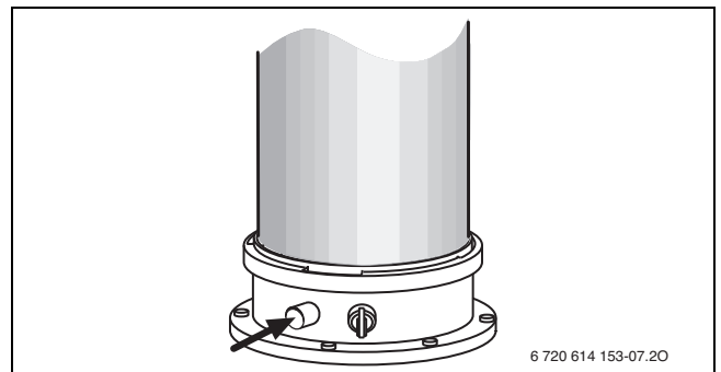
Мал. 40 Вимірювальний штуцер димових газів
