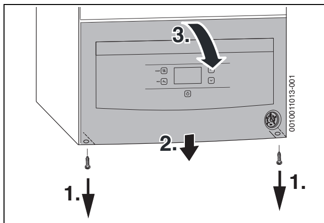
Мал. 23 Відкидання системи керування вниз
