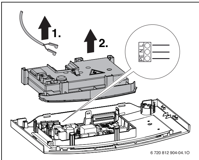
Мал. 30 Заміна мережевого кабелю
