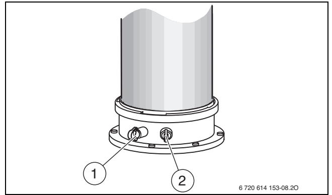
Мал. 44 Вимірювальний штуцер димових газів і штуцер для вимірювання повітря для горіння
