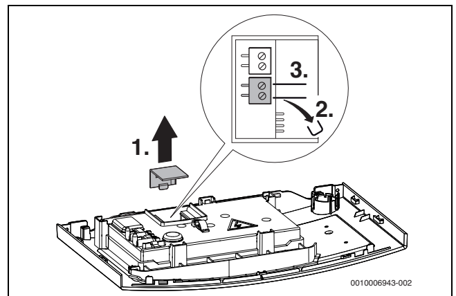
Мал. 28 Підключення системи керування
