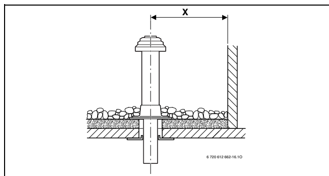
Мал. 5 Окремі розміри відстаней, плоский дах
