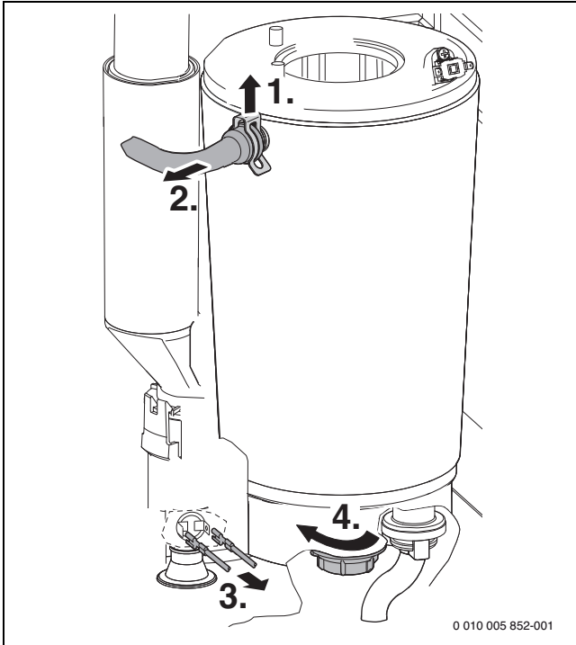
Мал. 65 Від'єднання труби лінії подачі та зняття кабелю
