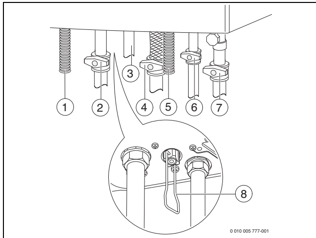
Мал. 26 Під'єднання з боку газо- та водопроводу (приладдя)
