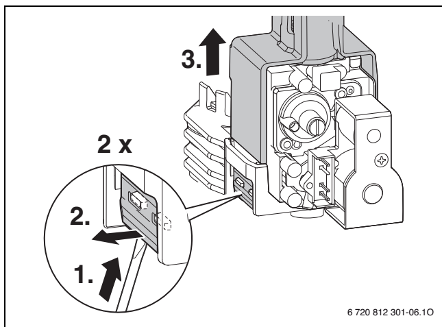
Мал. 62 Демонтаж газової арматури
