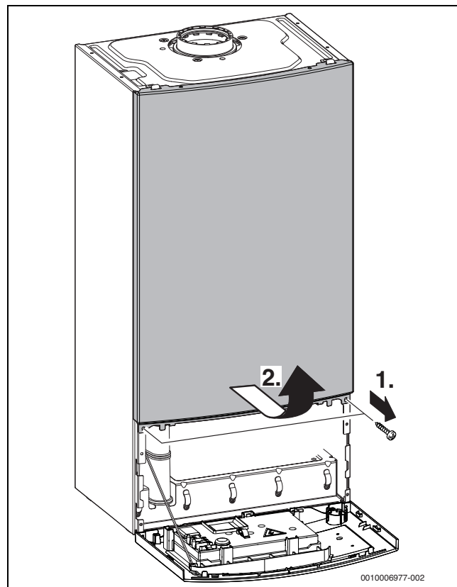
Мал. 25 Демонтаж передньої обшивки
