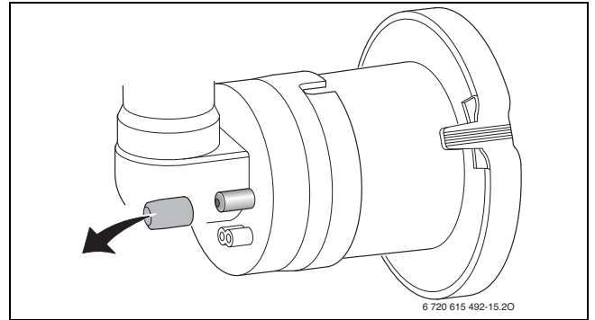
Мал. 45 Штуцер для вимірювання на змішувальній камері
