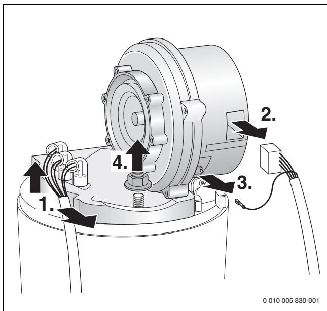
Мал. 47 Виймання вентилятора
