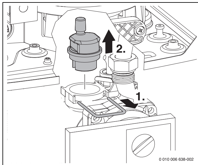
Мал. 59 Демонтаж автоматичного повітровідокремлювача
