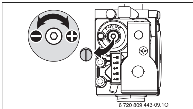
Мал. 42 Видалення пломби на газовій арматурі
