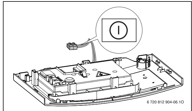
Мал. 31 Зовнішній комутаційний контакт, без потенціалу
