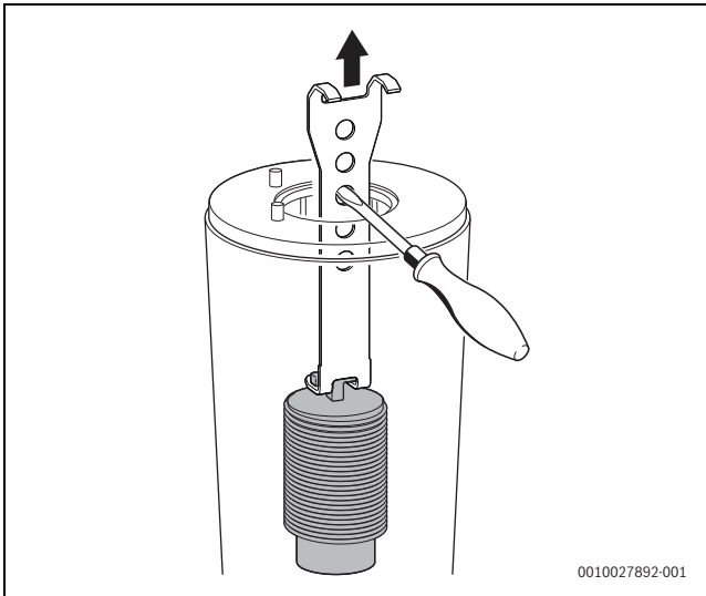
Мал. 54 Виймання нижнього елемента теплообмінника, що служить для оптимізації розподілювання тепла
