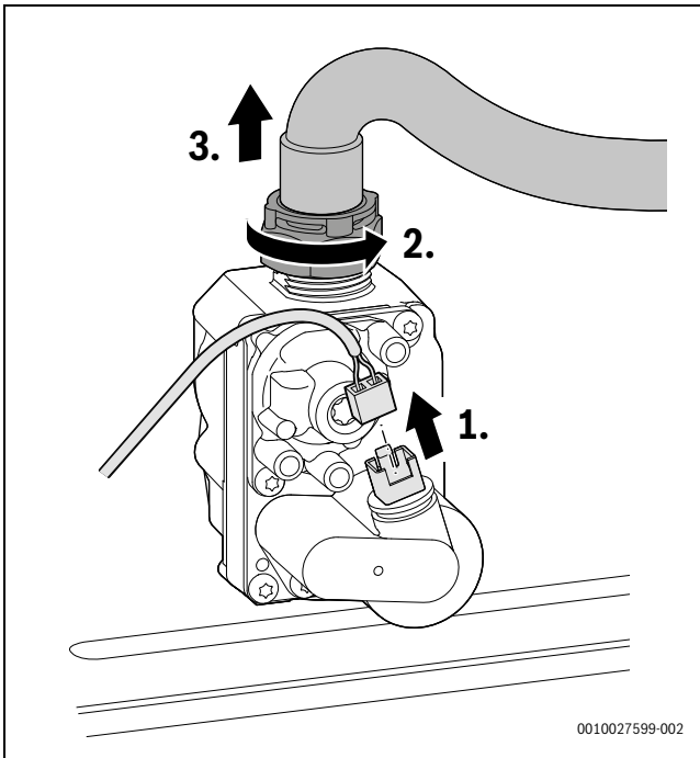
Мал. 67 Витягніть штекер газової арматури та зніміть накидну гайку разом з газовим шлангом
