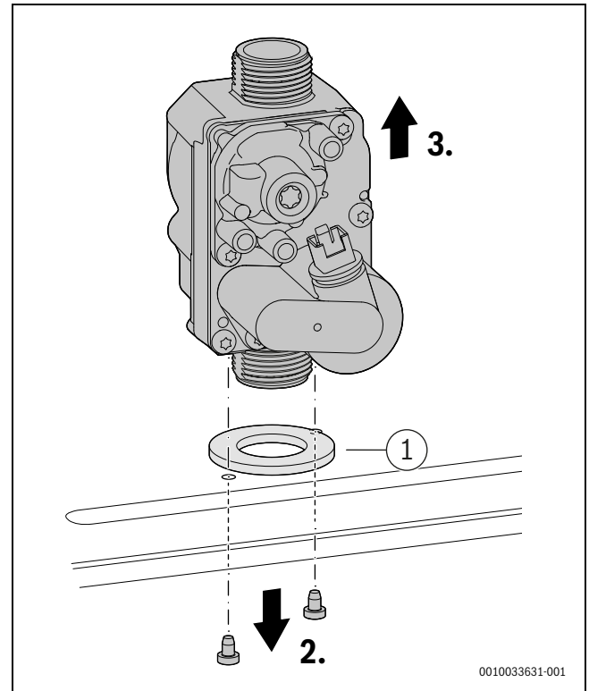
Мал. 70 Демонтаж газової арматури
