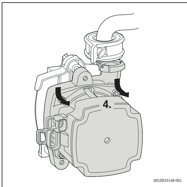
Мал. 65 Знімання насоса опалювального контуру
