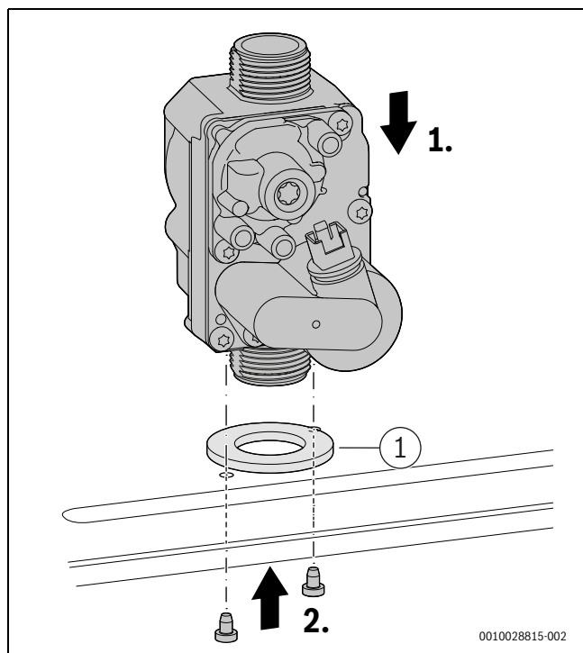
Мал. 71 Монтаж газової арматури
