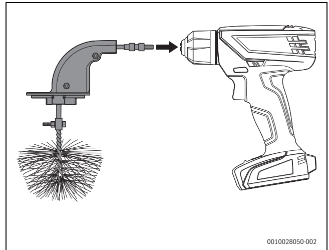
Мал. 56 З'єднайте щітку з акумуляторним шуруповертом
