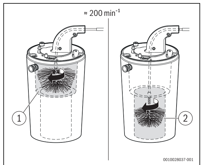
Мал. 57 Чищення котлового блоку, який включає камеру згоряння і теплообмінник (200 об/хв, тільки при правосторонньому обертанні)
