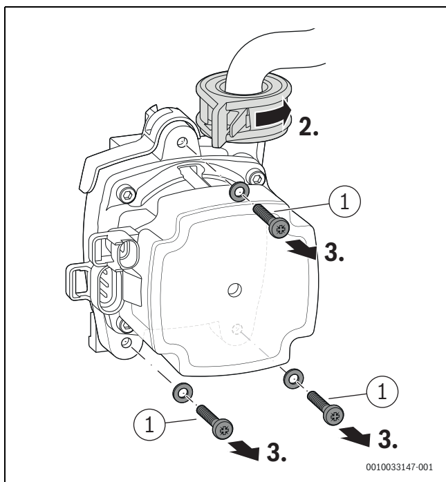
Мал. 64 Розблокуйте насос опалювального контуру та зніміть гвинти
