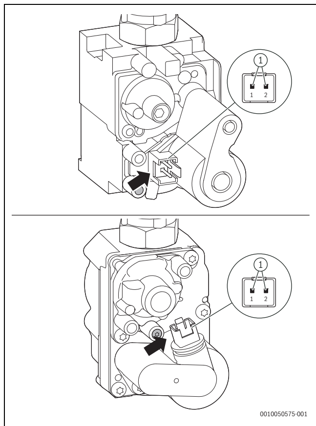
Мал. 47 Точки вимірювання на газовій арматурі
