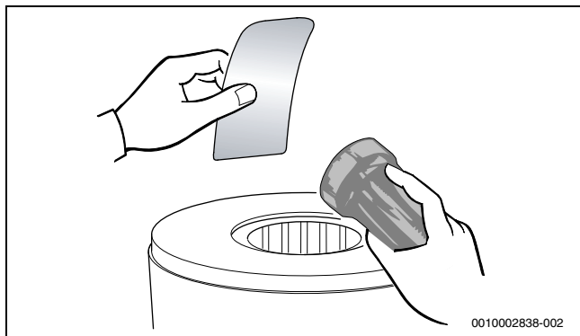
Мал. 59 Перевірка котлового блока, який включає камеру згорання і теплообмінник, на наявність відкладень
