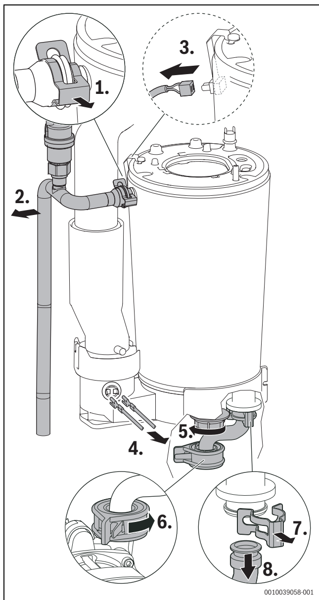
Мал. 61 Від'єднання труби лінії подачі, зняття кабелю та зняття труби зворотної лінії
